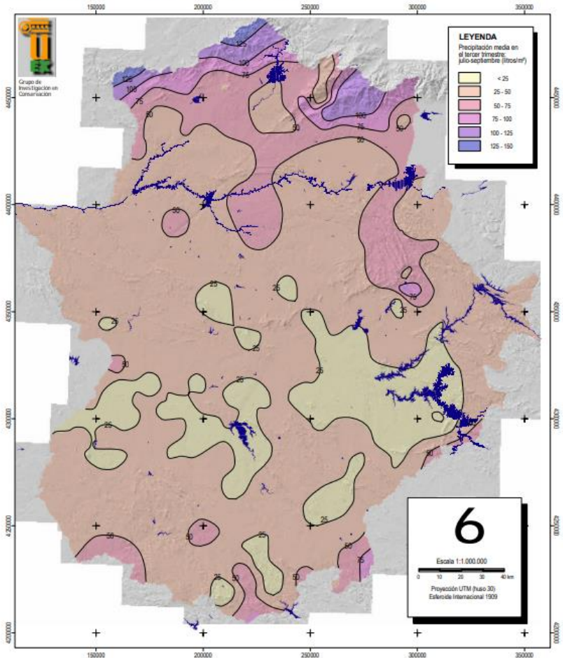
Precipitación media en el periodo julio-septiembre (litros/m 2 )
