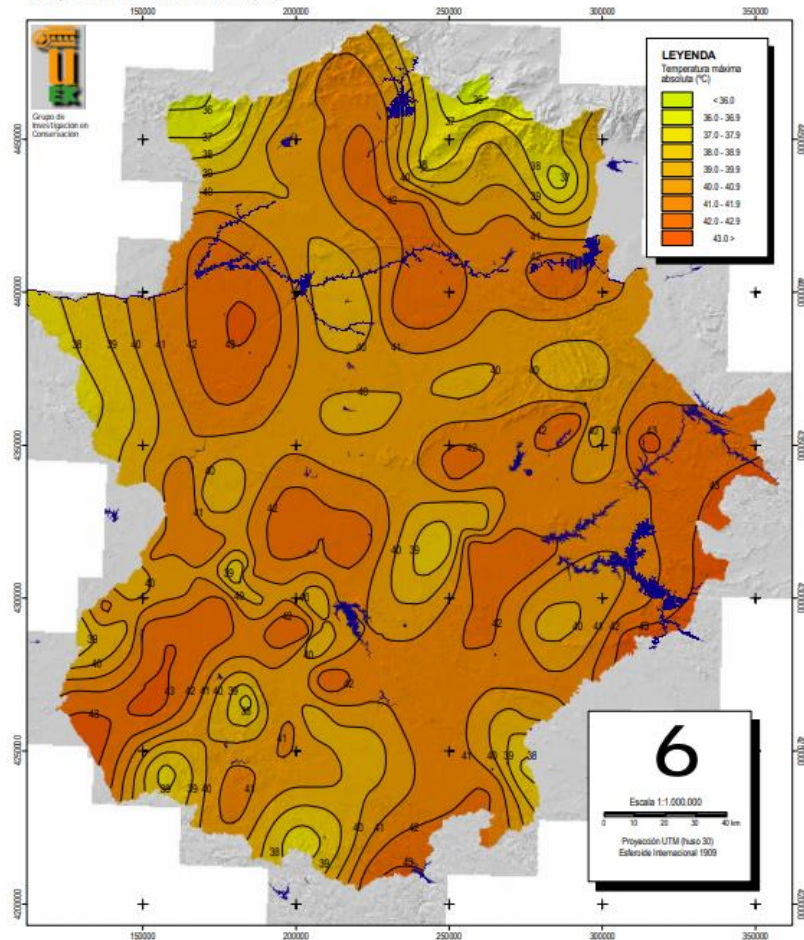
Temperatura máxima absoluta (°C)
